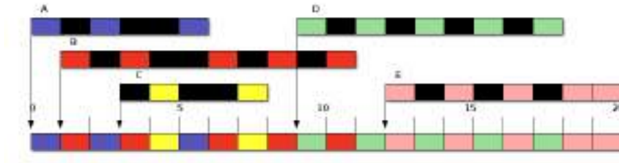
Figura 4.7: Ronda (Round Robin).
