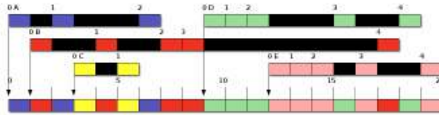
Figura 4.13: Retroalimentación multinivel (FB) básica.
