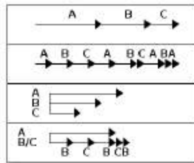
Figura 2.6: Esquema de la ejecución de tres procesos en un sistema secuencial, multiprogramado, multiprocesado, e híbrido.
