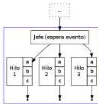
Figura 3.2: Patrón de hilos jefe/trabajador.
