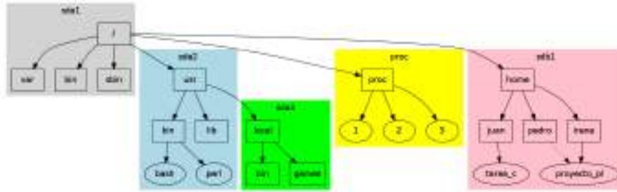
Figura 6.10: Árbol formado del montaje de sda1 en la raíz, sda2 como /usr , sdb1 como /home , y el directorio virtual proc .
