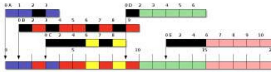
Figura 4.11: Ronda egoísta (SRR) con a = 2 y b = 1 .
