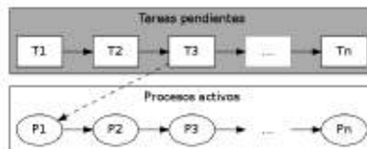
Figura 4.1: Planificador a largo plazo.
