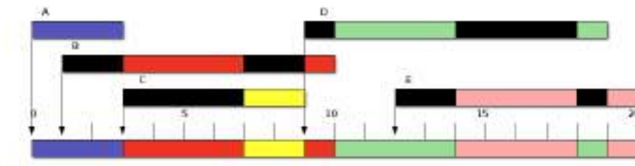
Figura 4.8: Ronda (Round Robin), con q = 4 .
