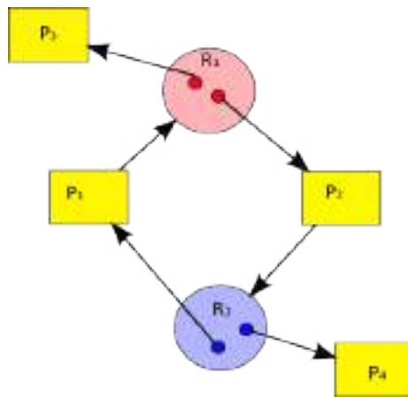
Figura 3.9: Al emplear categorías de recursos, un ciclo no necesariamente indica un bloqueo.
