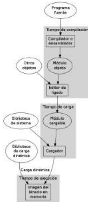
Figura 5.4: Proceso de compilación y carga de un programa, indicando el tipo de resolución de direcciones (Silberschatz, Galvin y Gagné 2010: 281).
