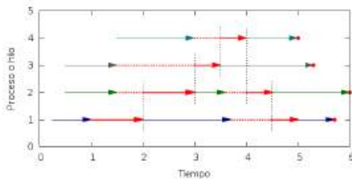
Figura 3.5: Sincronización: la exclusión de las secciones críticas entre varios procesos se protegen por medio de regiones de exclusión mutua . La figura ilustra varios procesos que requieren de una misma sección crítica; las flechas punteadas representan el tiempo que un proceso está a la espera de que otro libere el paso para dicha sección, y las punteadas verticales indican la transferencia del candado .
