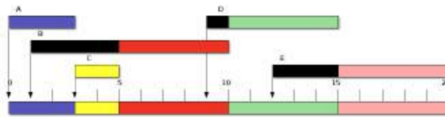
Figura 4.9: El proceso más corto a continuación (SPN).
