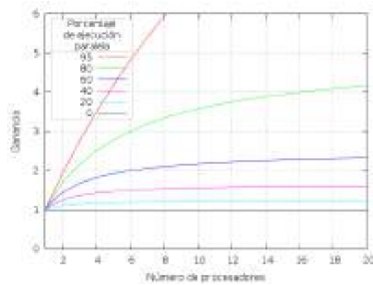
Figura 2.10: Ganancia máxima al paralelizar un programa, ilustrando los límites que impone la Ley de Amdahl.
