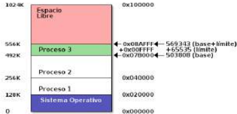
Figura 5.1: Espacio de direcciones válidas para el proceso 3 definido por un registro base y uno límite.
