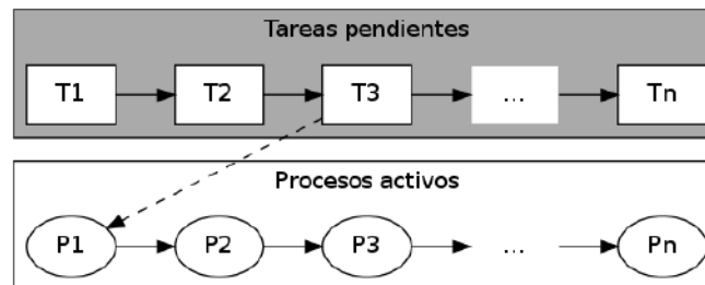
Figura 5.1: Planificador a largo plazo
