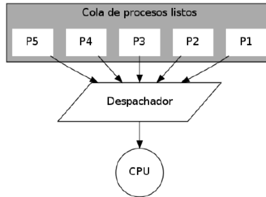
Figura 5.3: Planificador a corto plazo, o despachador
