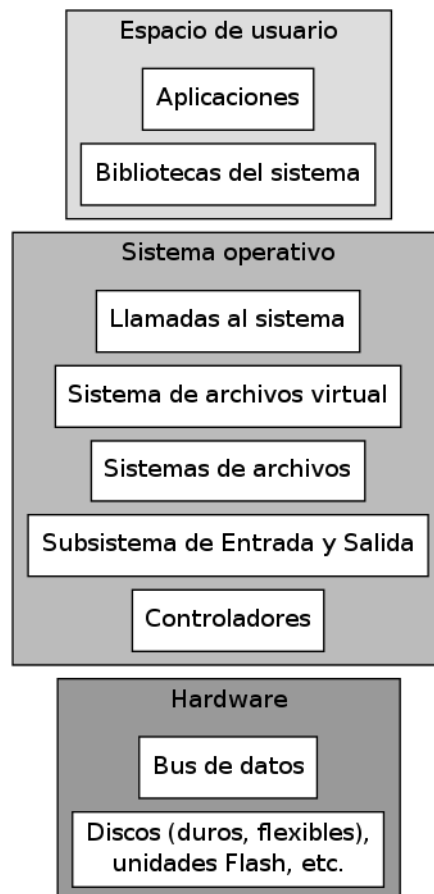
Figura 7.1: Capas de abstracción para implementar los sistemas de archivos
