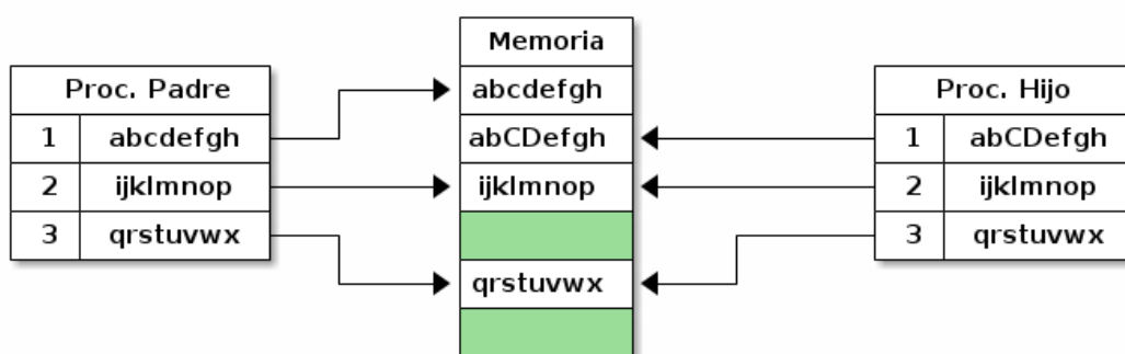
Figura 6.14: Cuando el proceso hijo modifica información en la primer página de su memoria, se crea como una página nueva.
