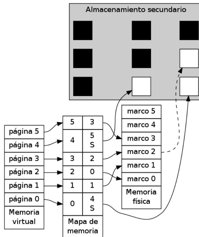
Figura 6.15: Esquema general de la memoria, incorporando espacio en almacenamiento secundario, representando la memoria virtual
