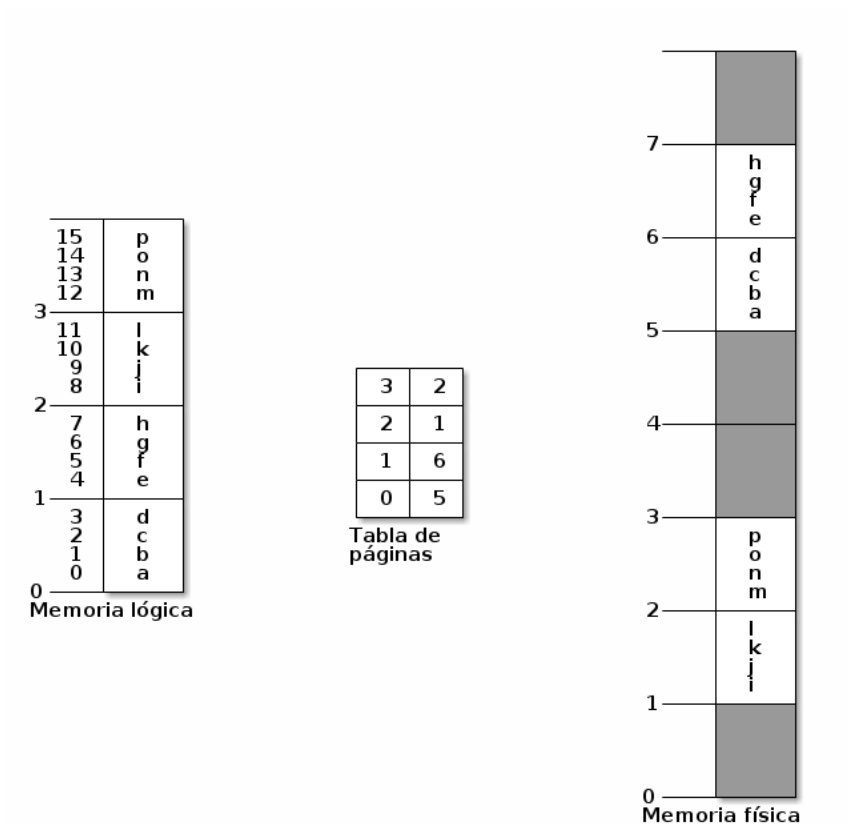
Figura 6.9: Ejemplo (minúsculo) de paginación, con un espacio de direccionamiento de 32 bytes y páginas de 4 bytes
